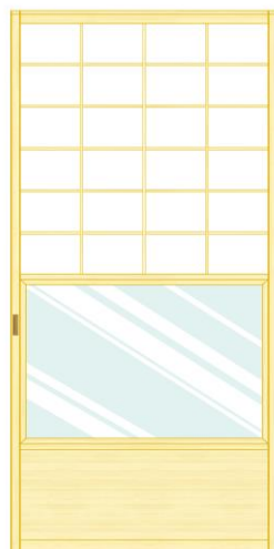
HRC-505 腰板中硝子障子
